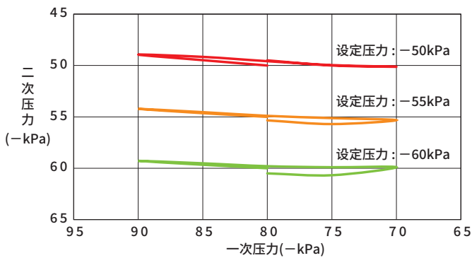
压力特性图
