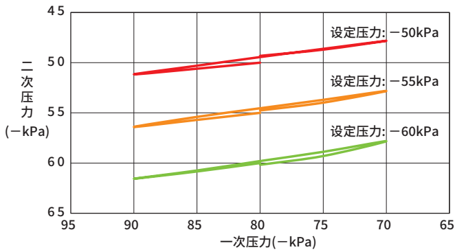
压力特性图
