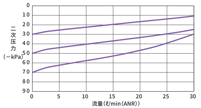
流量特性图
