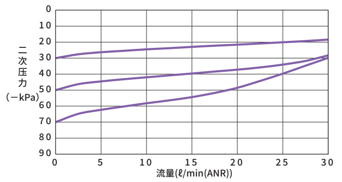
流量特性图
