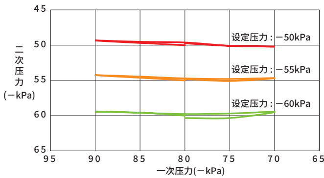
压力特性图
