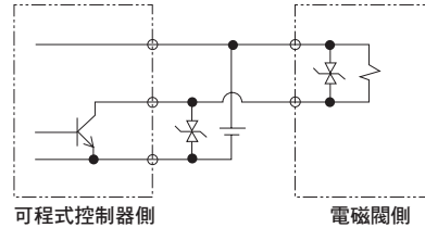
〈輸出電晶體保護迴路 併設範例2〉
