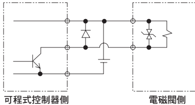
〈輸出電晶體保護迴路 併設範例1〉
